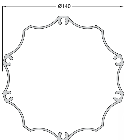
Código: 67 PESO/WEIGHT 3153 gr/m COLUMNA 140x140 COLUMN 140x140
