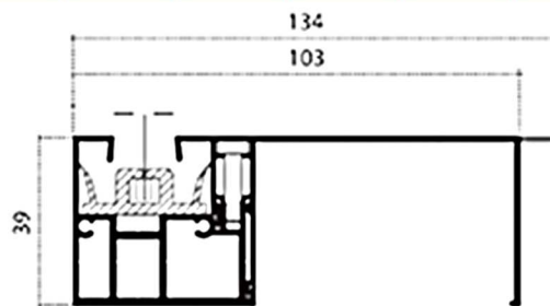
GUÍA OCULTA HIDDEN GUIDE
