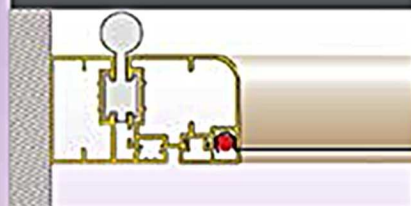
MARCO PERFIL ESTÁNDAR "L" FRAME PROFILE "L" STANDARD
