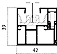
GUÍA ESTÁNDAR STANDARD GUIDE
